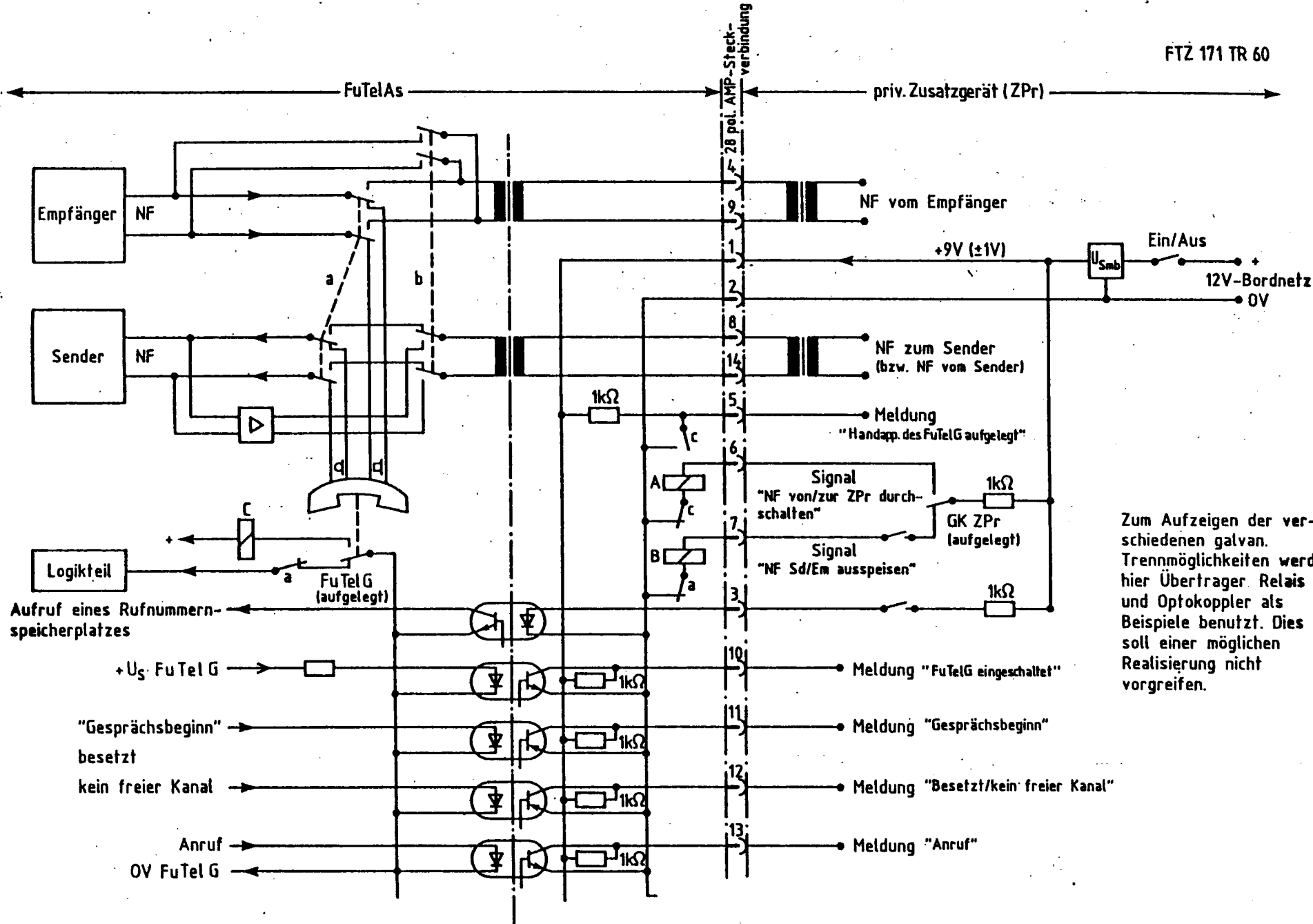
Bild 8.3 Prinzipielle Funktionsschaltung der Schnittstelle für Zusatzgeräte an FuTel G
