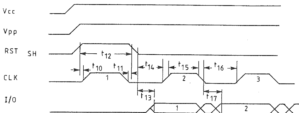
Bild 1: Reset der Chipkarte und Auslesen des Speicherinhalts
